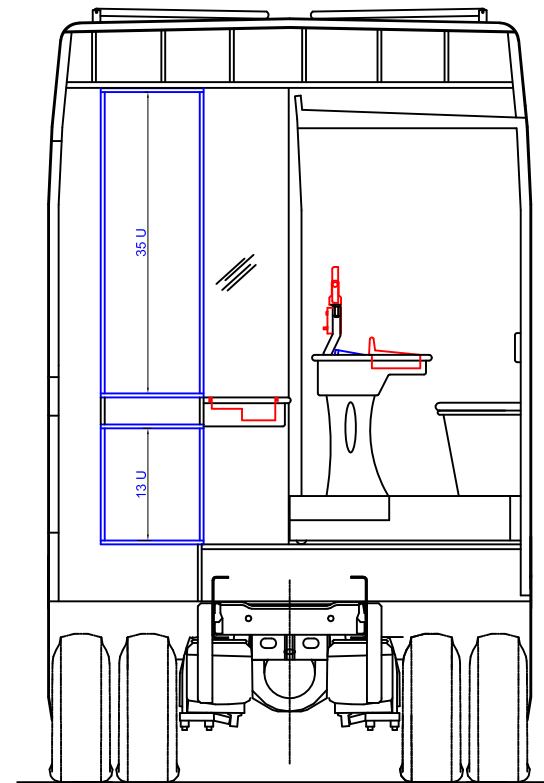
SECCION C-C (PETACA CERRADA)
