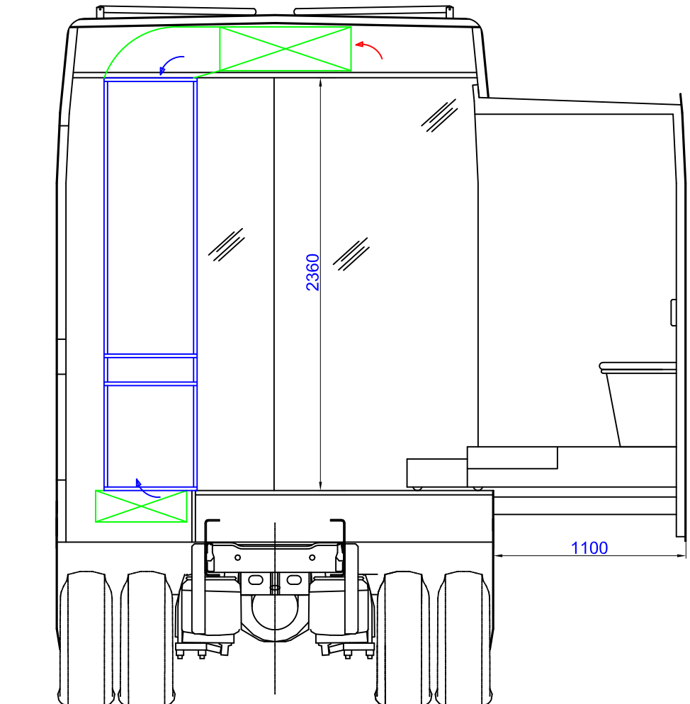
SECCION H-H
