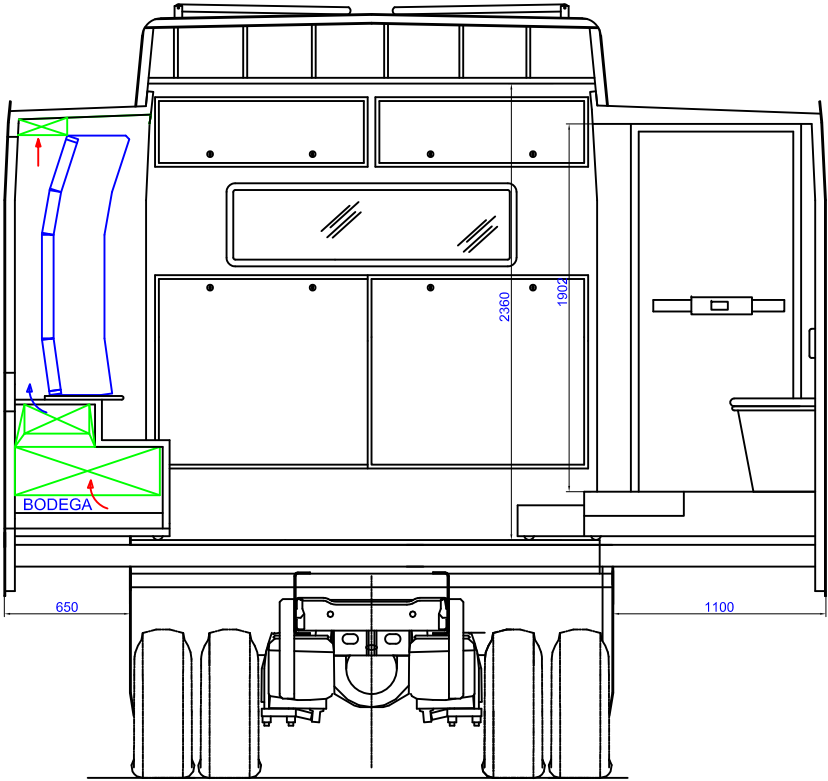
SECCION I-I
