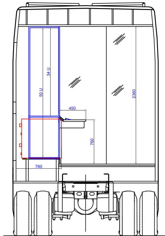
SECCION B-B (C. TÉCNICO)
