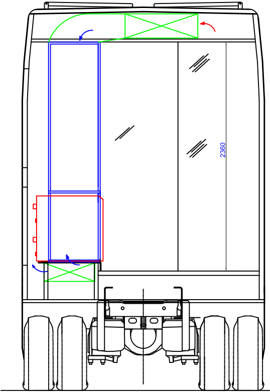
SECCION G-G
