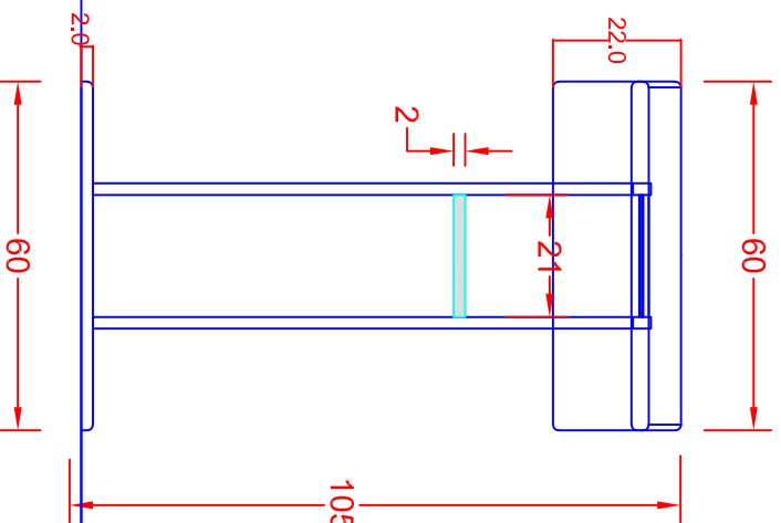
ALZADO FRONTAL
