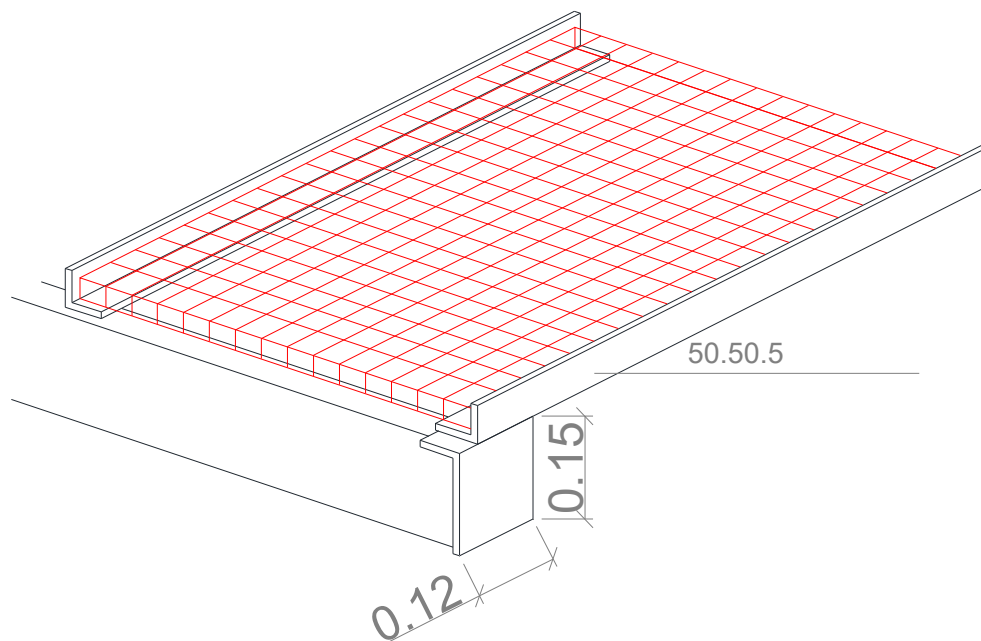
Figura 1. Perspectiva Pasarela NNEE Planta 2ª Edificio Nuevos Estudios
