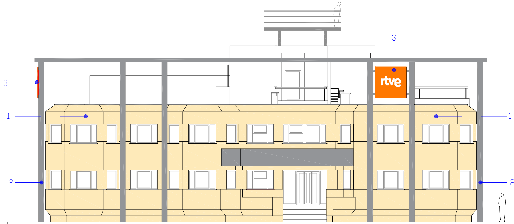
ALZADO
