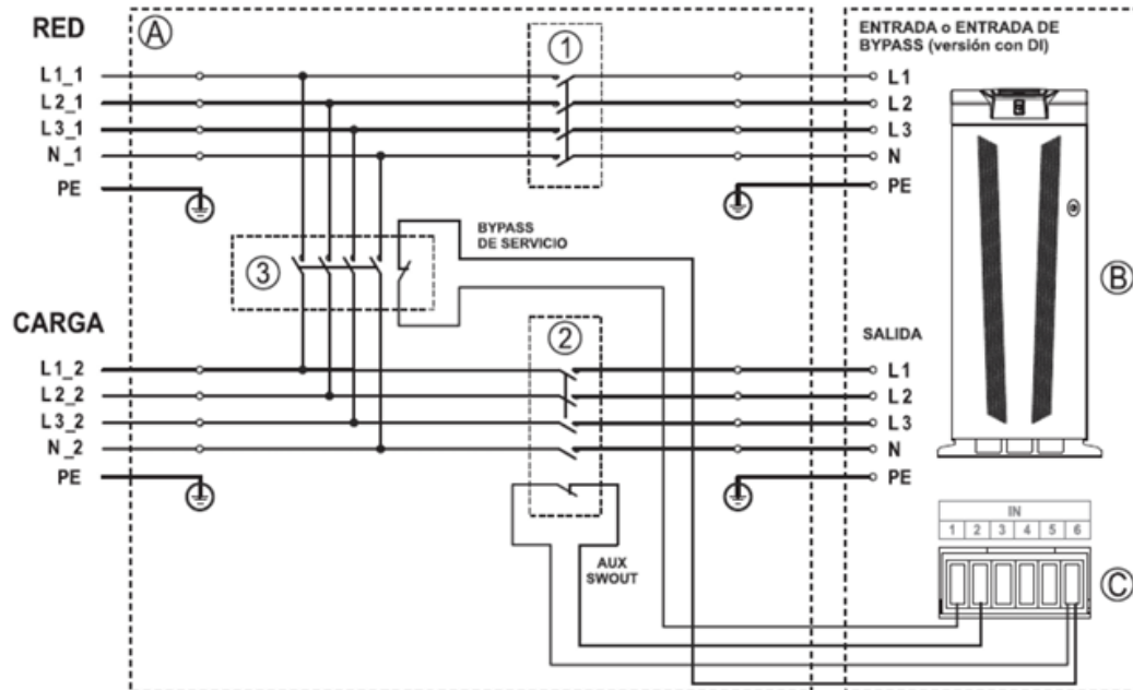
DIAGRAMA DE LA INSTALACIÓN DEL BYPASS DE MANTENIMIENTO (MODELO S3T)
