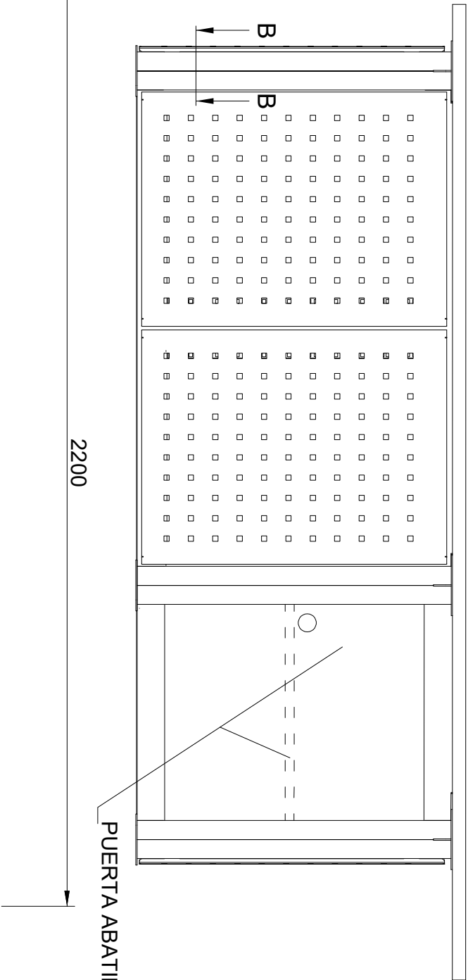
VISTA POSTERIOR
