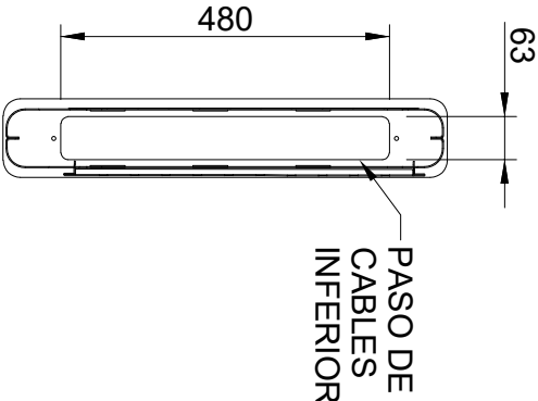
CORTE B-B
