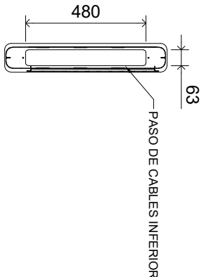
CORTE B-B
