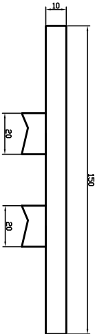
CHAPAS SUPERIORES DE CARRIL Y UNIÓN DE PERFILES
